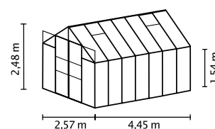
URANUS 11500
