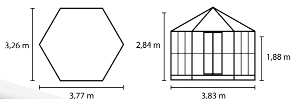
HERA 9000
