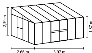
HELENA 10200
