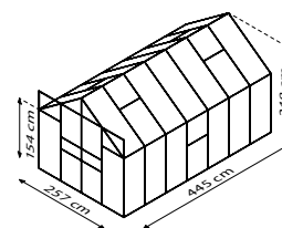
JUPITER 11500
