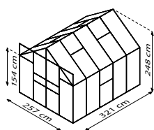
JUPITER 8300
