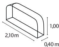
KAMINHOLZUNTERSTAND QUER
